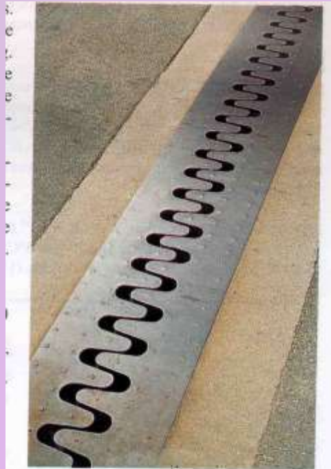
17.12 Los dientes de una articulación de expansión de un puente. Se requieren estas articulaciones para dar cabida a los cambios de longitud resultado de la expansión térmica.
